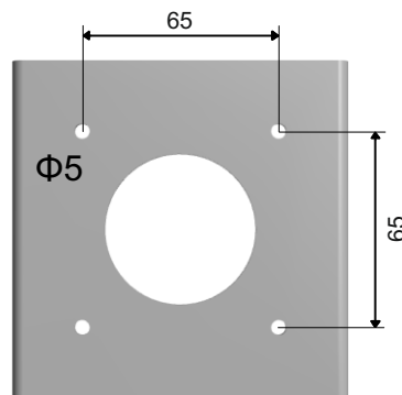
podstawa oprawy
